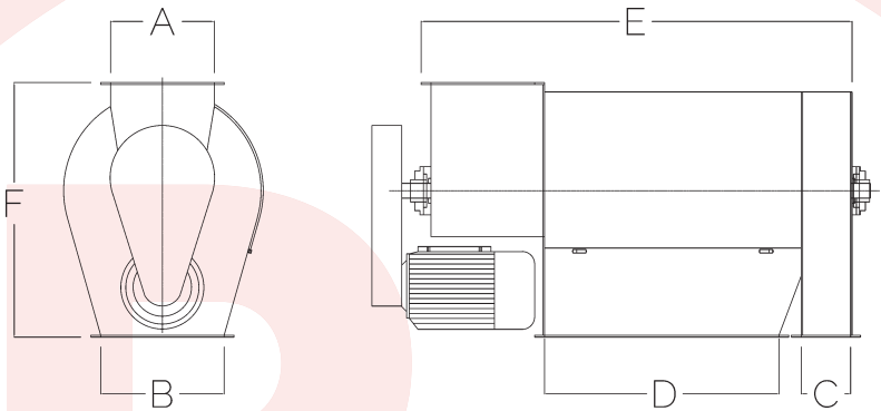
MEDIDAS GENERALES (mm) / GENERAL MEASUREMENTS (mm) / MESURES GÉNÉRALES (mm)
